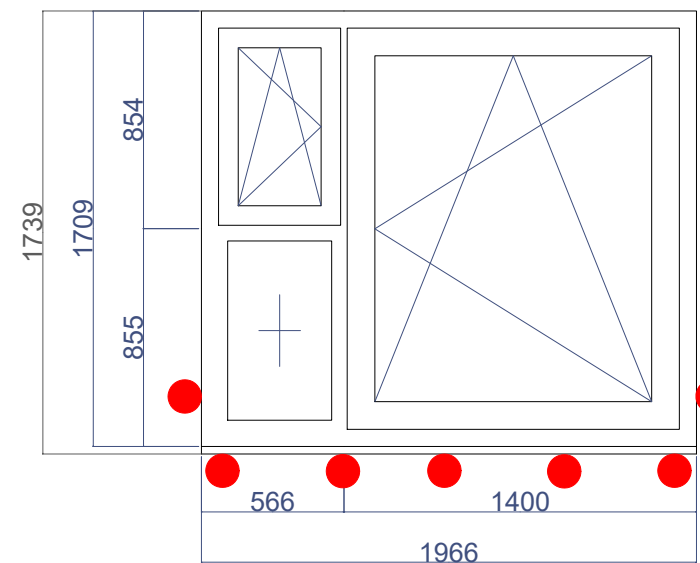
Innenansicht M 1:30
